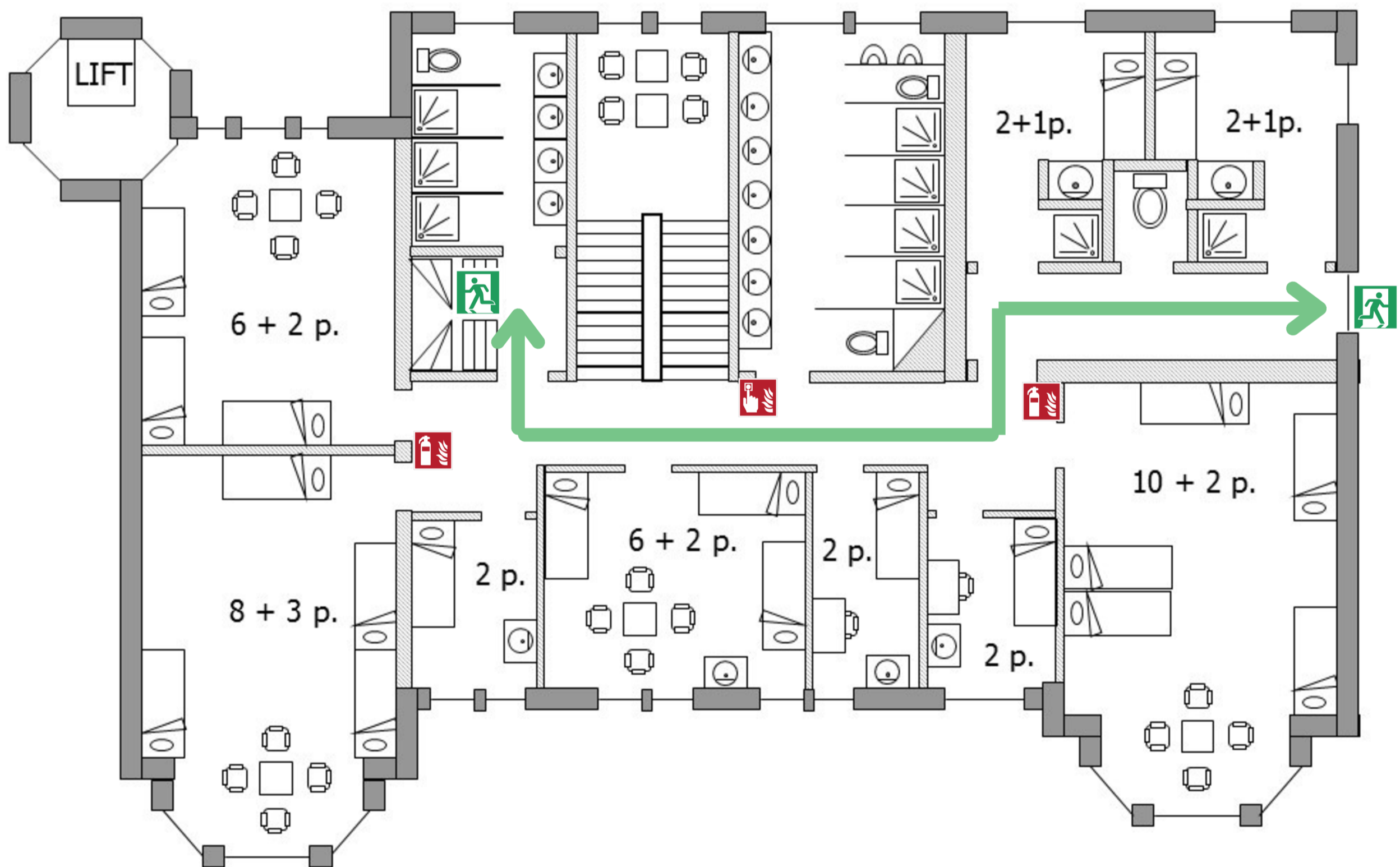
Eerste verdieping
