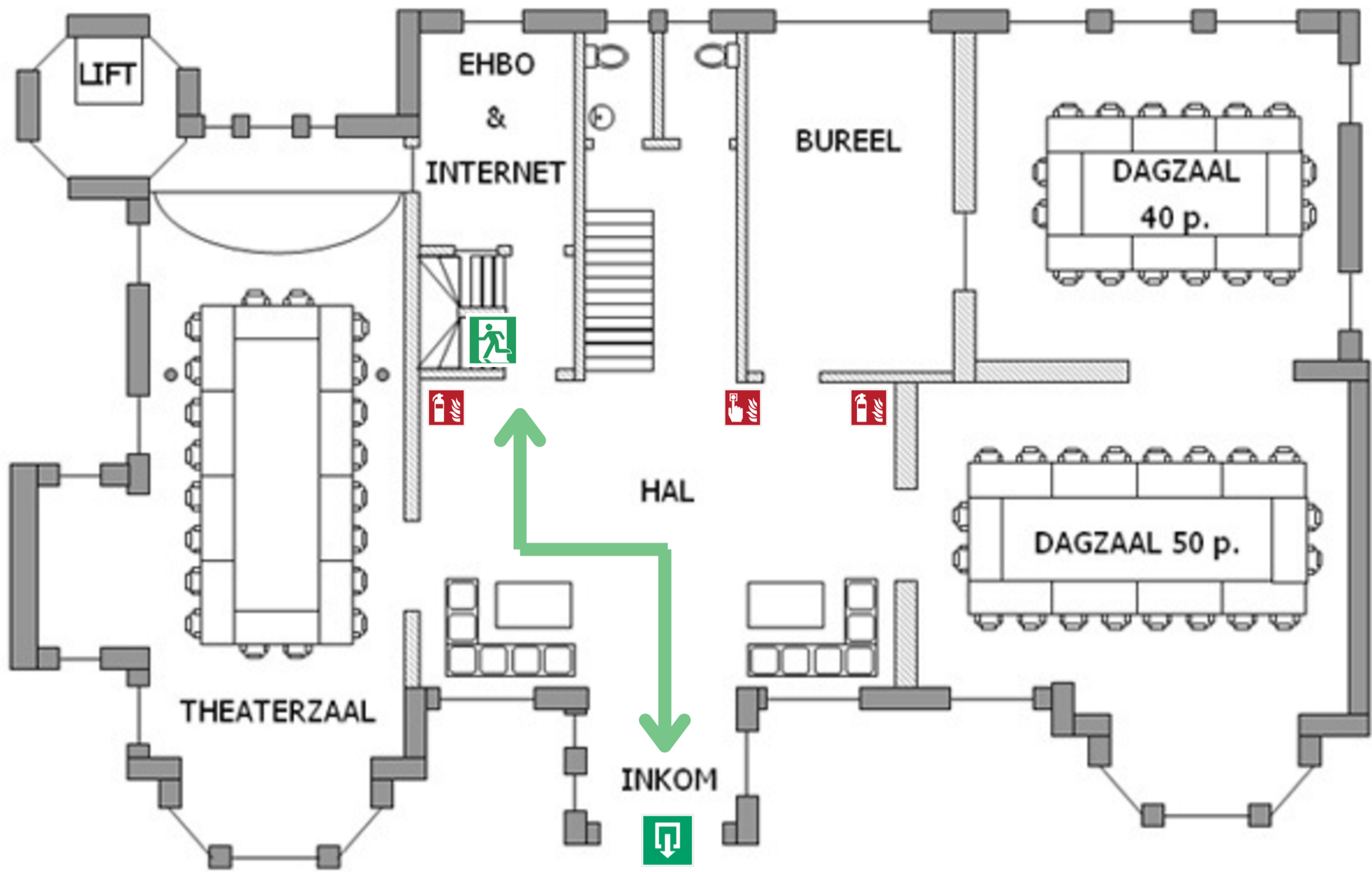
Gelijkvloers
